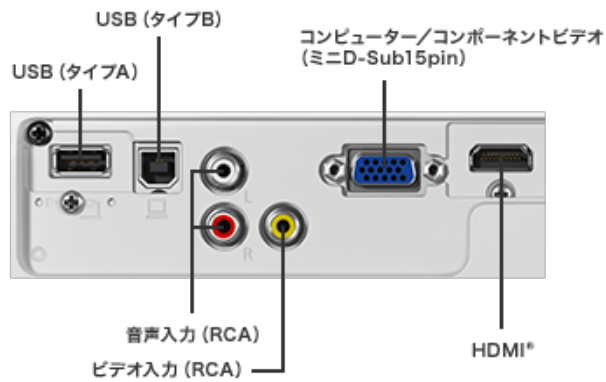
プロジェクター背面 EPSON EB-X06
